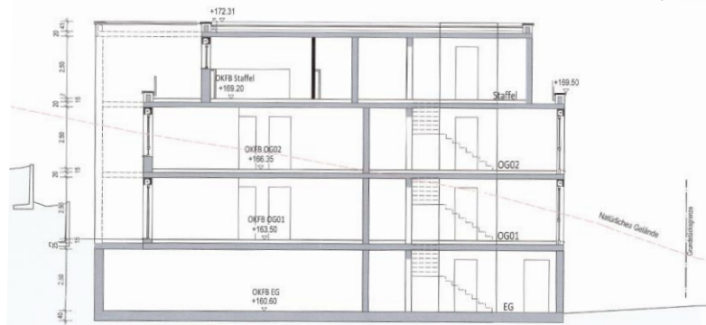
Schnitt A-A
