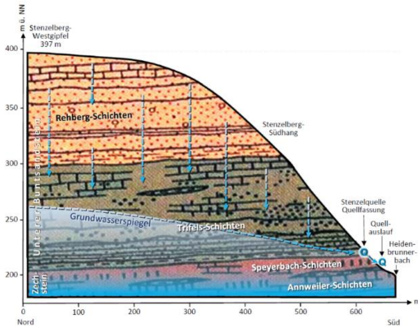
Abbildung 51: Schematisches hydrogeologisches Profil einer Schichtquelle im Stadtwald (Stenzelquelle im Heidenbrunner Tal) 122
