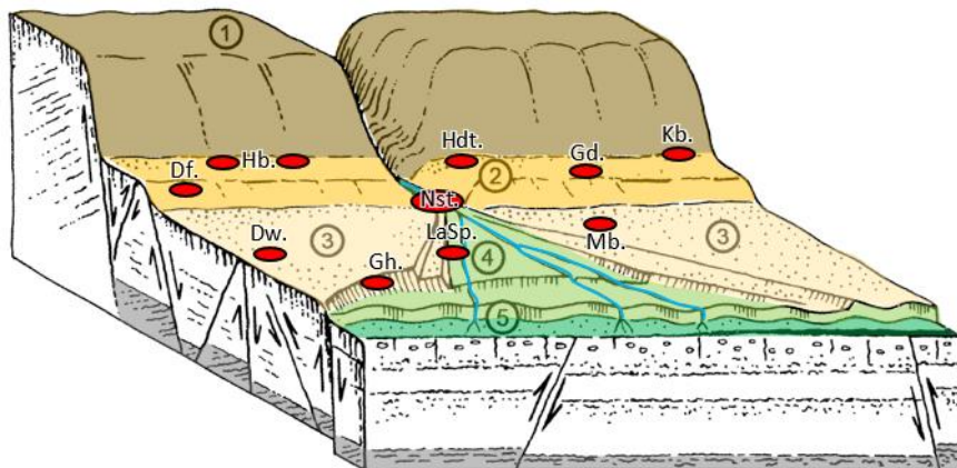
Abbildung 35: Relief und Tektonik: Schematisches Blockbild des Stadtgebiets von Südosten 95
