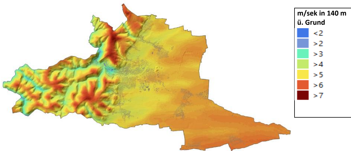
Abbildung 27: Windgeschwindigkeiten in Abhängigkeit von der Topografie in 140 m über Grund 81
