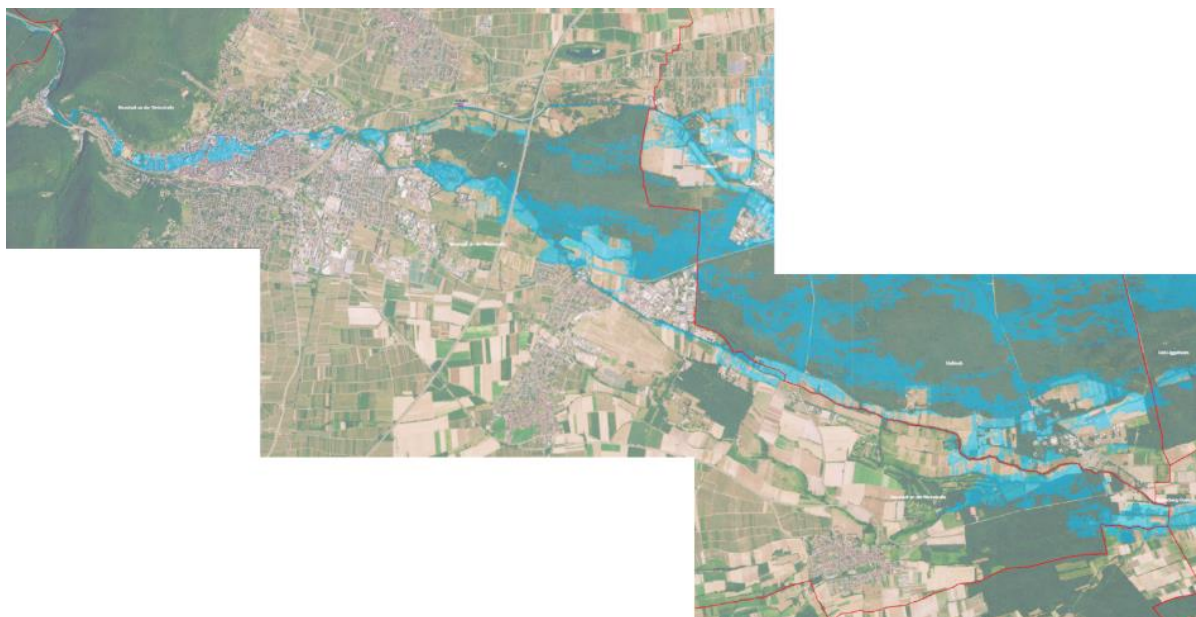
Abbildung 66: Aktualisierte Hochwassergefahrenkarte (HWGK) für das Speyerbach-Rehbach-System im Stadtgebiet von Neustadt bei Extrem-Hochwasser (HQextrem), 2021 143
