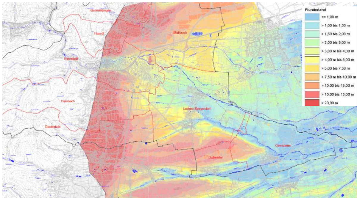
Abbildung 48: Grundwasser-Flur-Abstand in der Rheinebene 119
