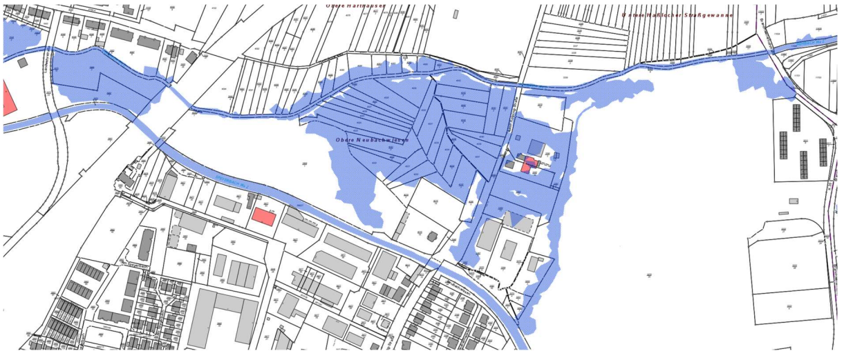
Abbildung 1 Überflutungsfläche HQ100
