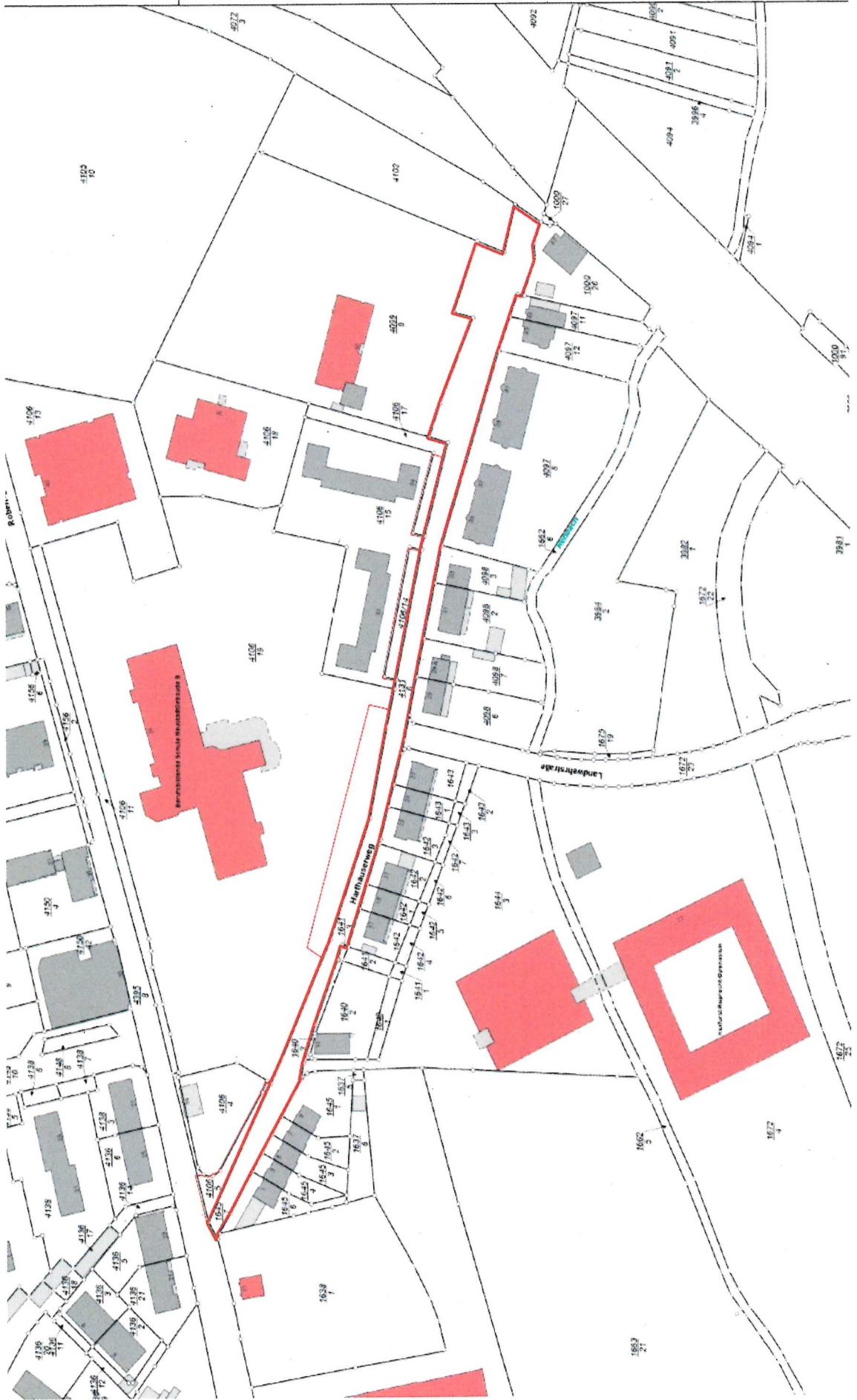
Lageplan Harthäuserweg, Flurstücks-Nr.: 4106/5 (teilw.), 4106/19 (teilw.), 4131/6, 4106/14, 4106/17 (teilw.)
